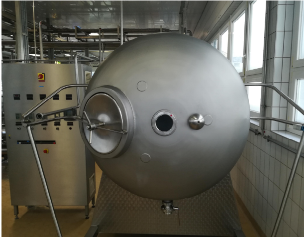
Butterfass zur diskontinuierlichen Herstellung
